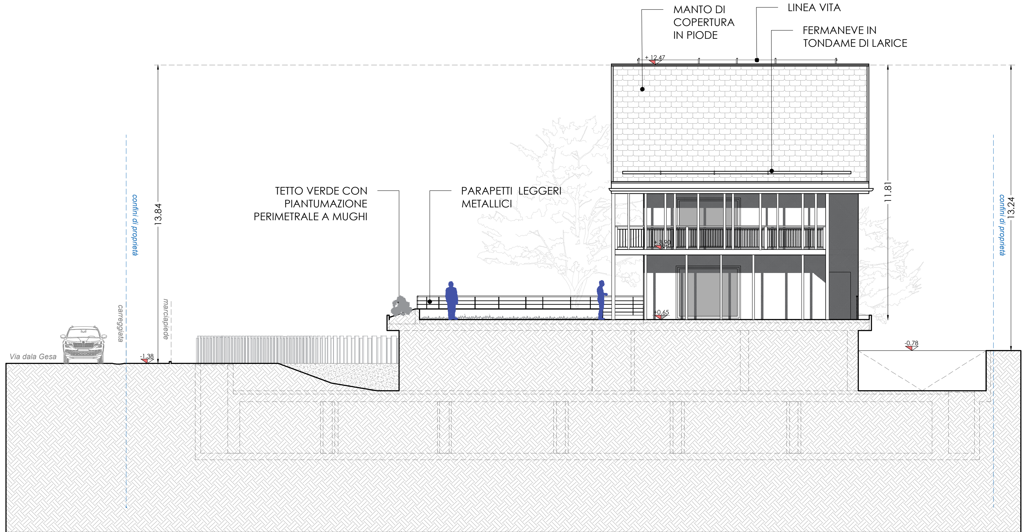
PROSPETTO NORD
