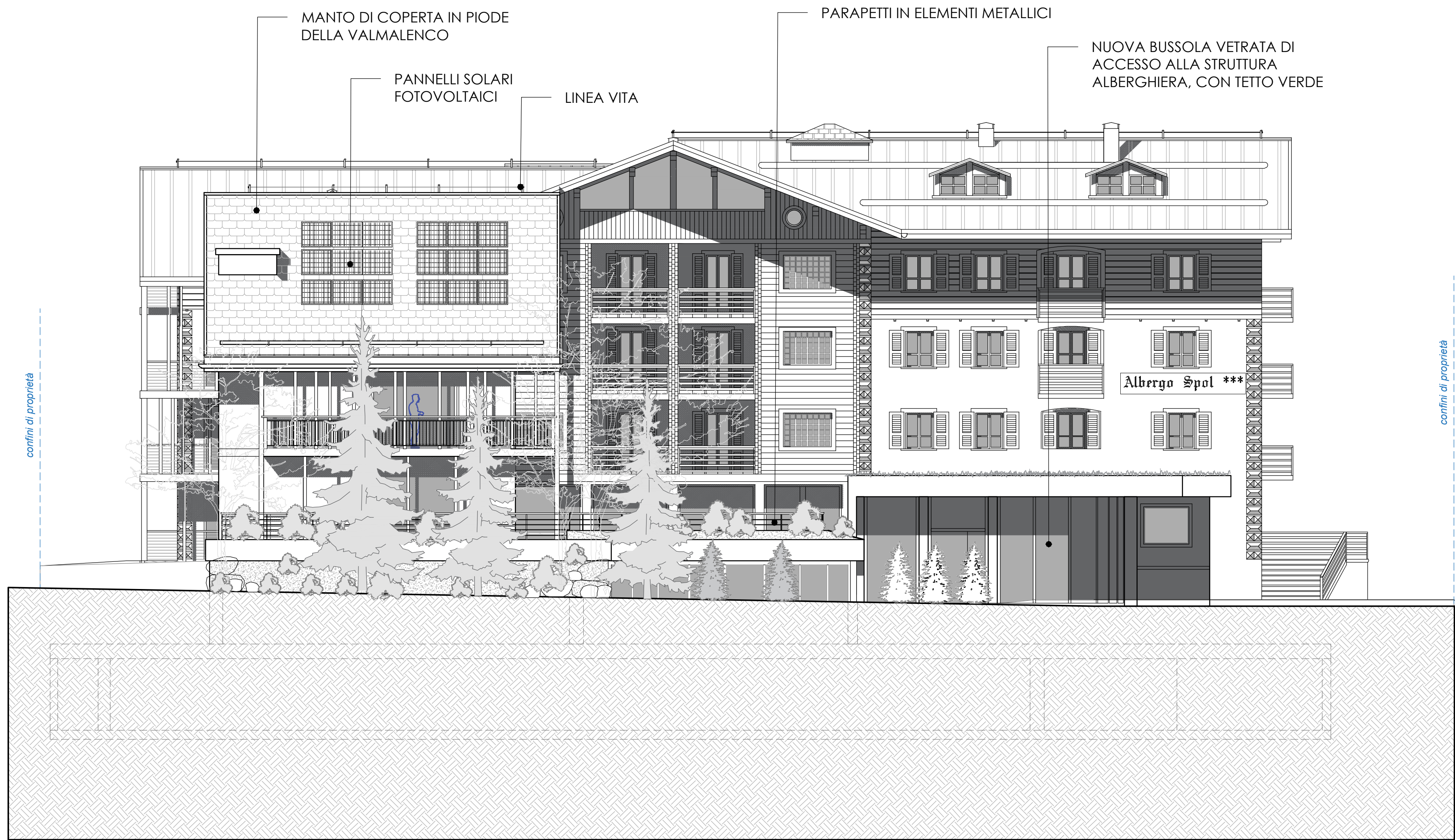
PROSPETTO SUD
