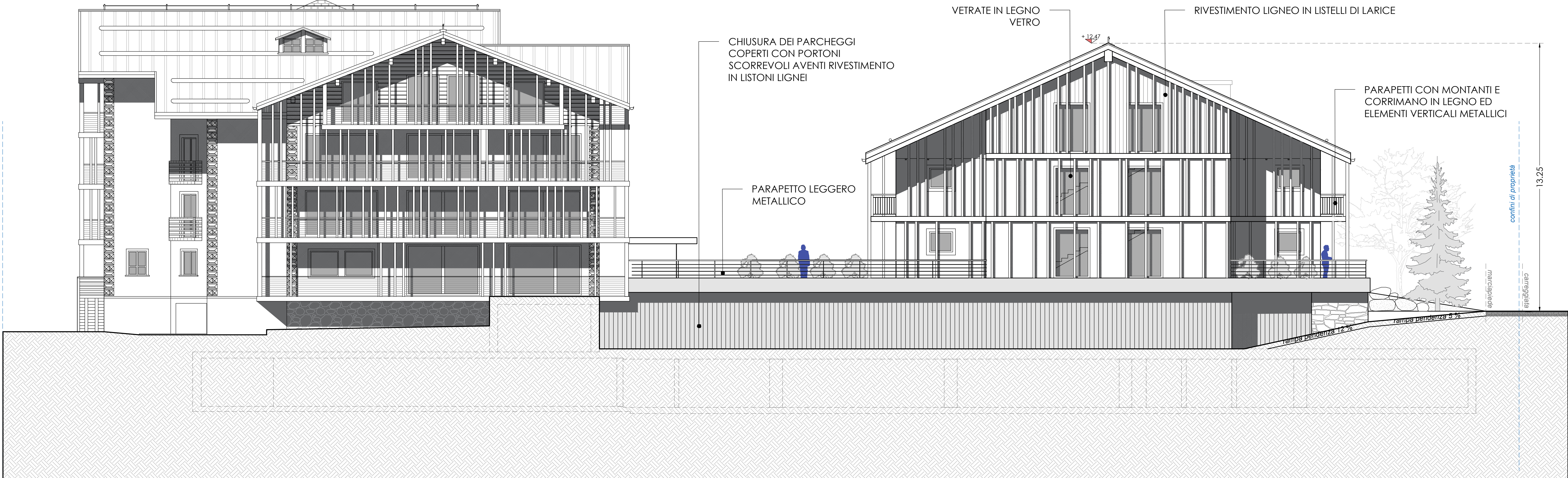
PROSPETTO OVEST
