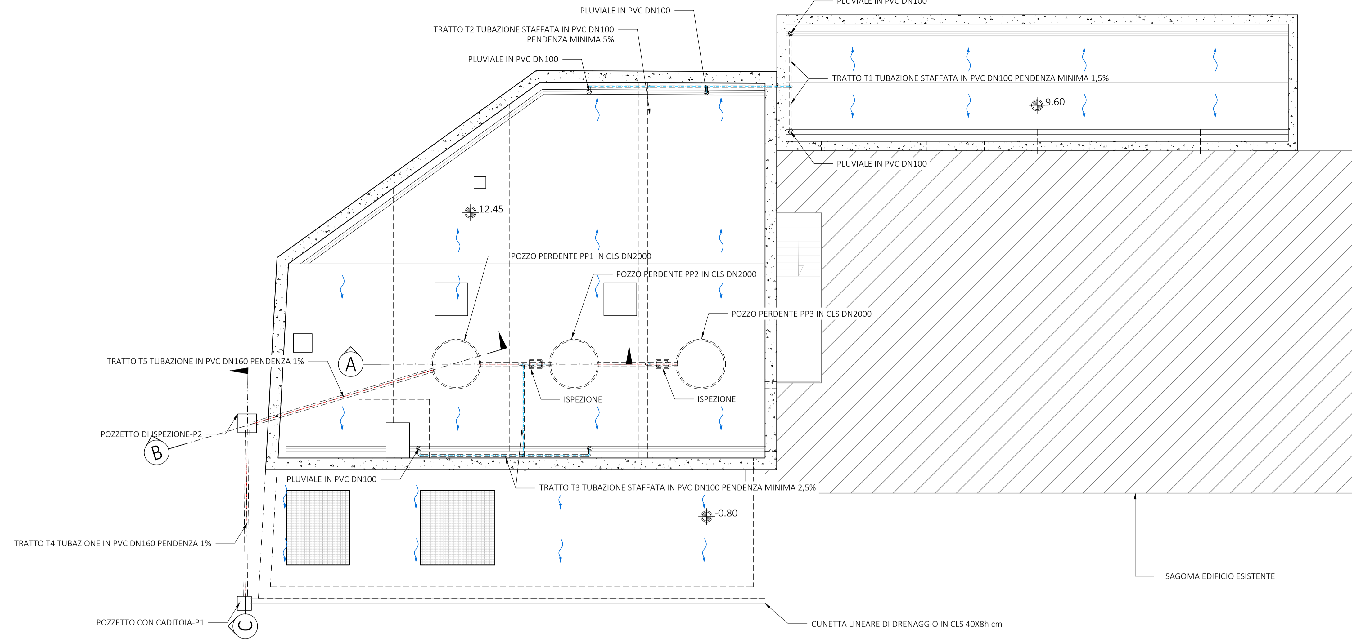
SCALA 1:100: PIANTE PIANO TERRA
