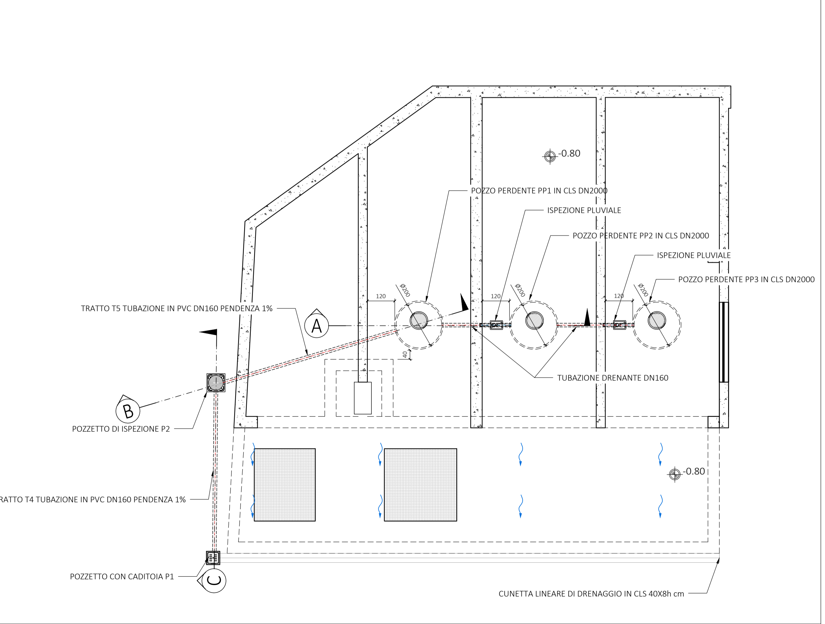
SCALA 1:100: PIANTE PIANO TERRA
