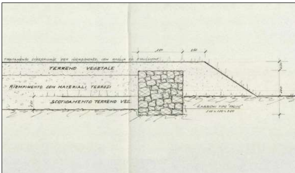
Fig. 3 – Sezione “tipo” dell’anello idraulico (estratto tavola progettuale “PARTICOLARI COSTRUTTIVI – anno 1987)
