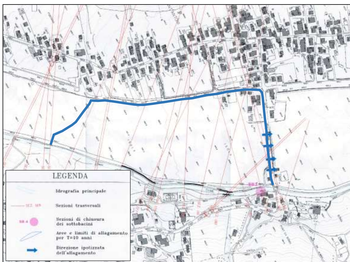
Fig. 7 – Area oggetto di esondazione con tempo di ritorno di 10 anni (estratto dalla tavola “MODELLAZIONE IDRAULICA – Planimetria aree di allagamento (T=10 anni)” dello “Studio idrologico ed idraulico” di riferimento)
