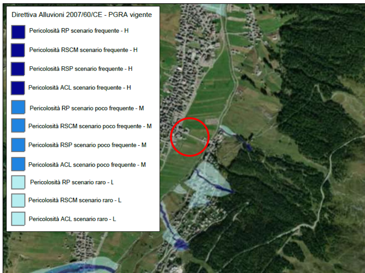
Fig. 5 – Stralcio carta Direttiva Alluvioni 2007/60/CE – PGRA Vigente – Pericolosità (fonte S.I.T. Regione Lombardia)
